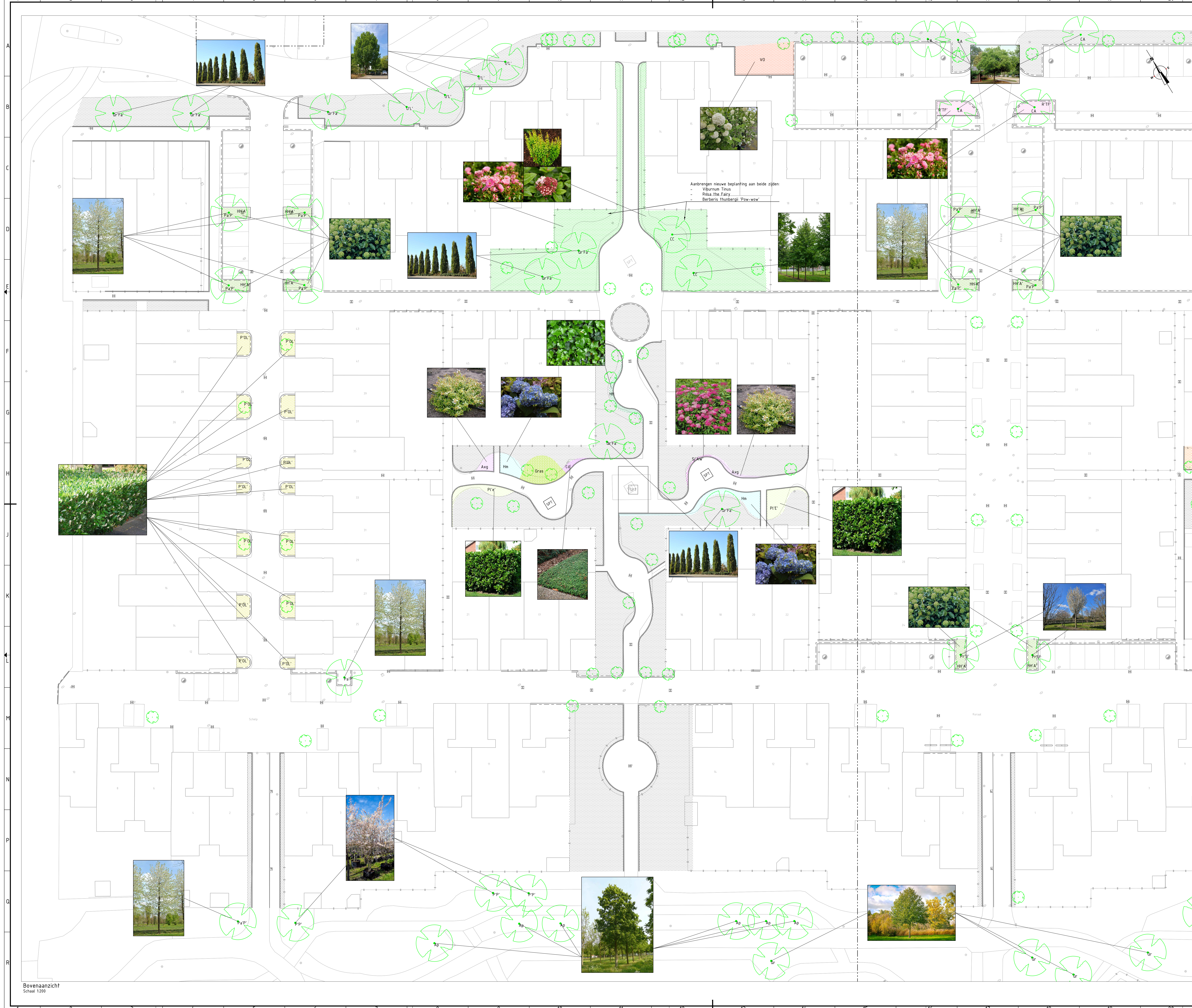
Situatie Schaal 1:5000
